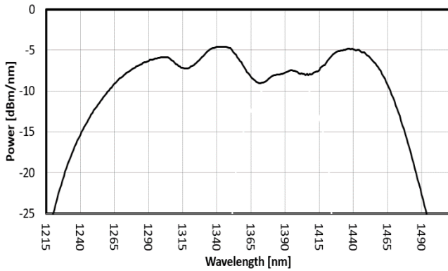
FIG. 1: ISB2 SPECTRUM
