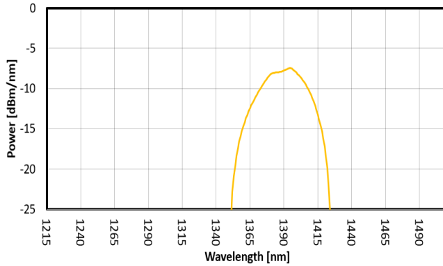
FIG. 3: SLED 2 SPECTRUM
