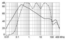
25A (FMAC-0932-2510)
